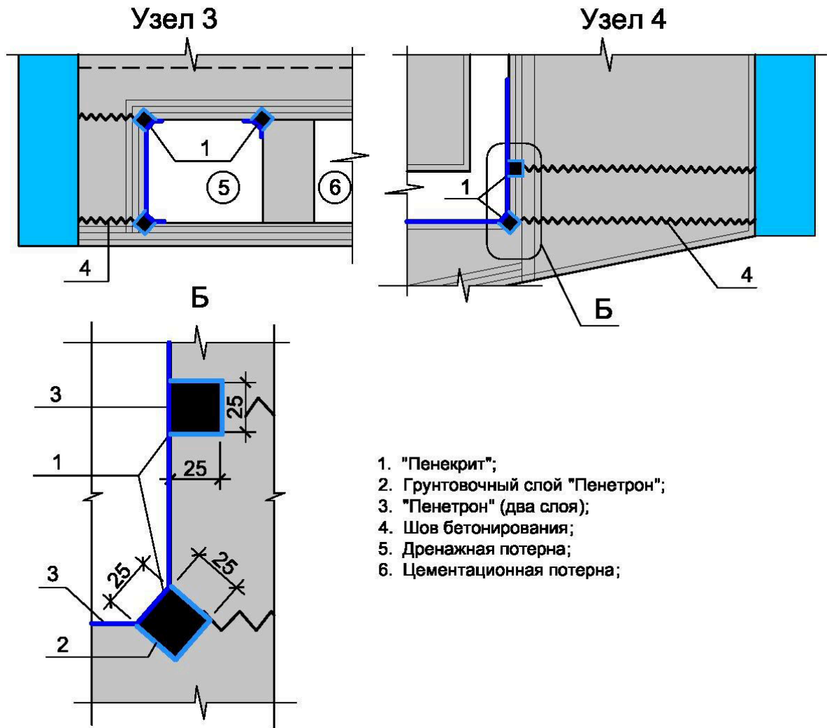
Рисунок 7.2.8 - Типовые узлы гидроизоляции в потернах, смотровых шахтах и соединительных коридорах (узлы 3 и 4 на рис. 7.2.7)
