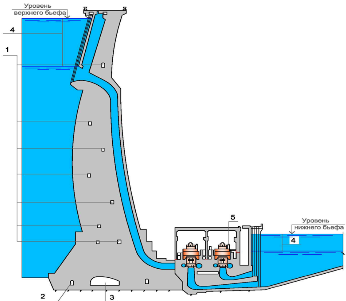
Рисунок 6.2.2 - Бетонная арочная плотина:
