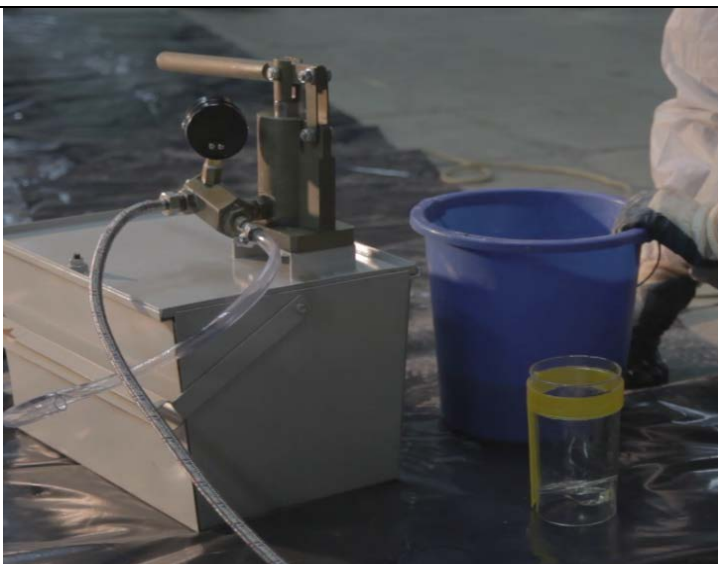
Рисунок 7.2.29 – Пробное смешивание компонентов
